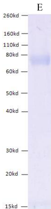
E: HA( \Delta TM)(H1N1)(A/Puerto Rico/8/1934)
